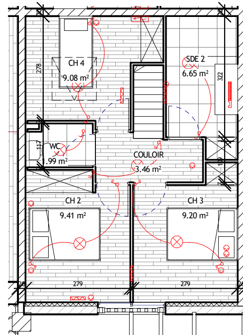
2 E311 Ech : 1 : 100
