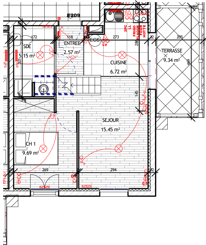
1 E 209 Ech : 1 : 100
