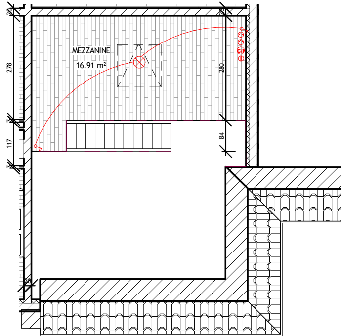
2 E309 Ech : 1 : 100
