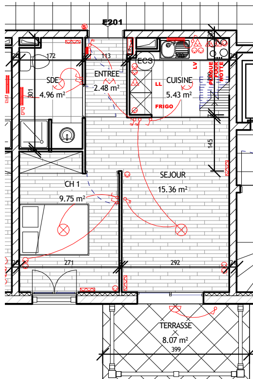
1 E 201 Ech : 1 : 100
