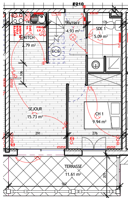
1 E 210 Ech : 1 : 100
