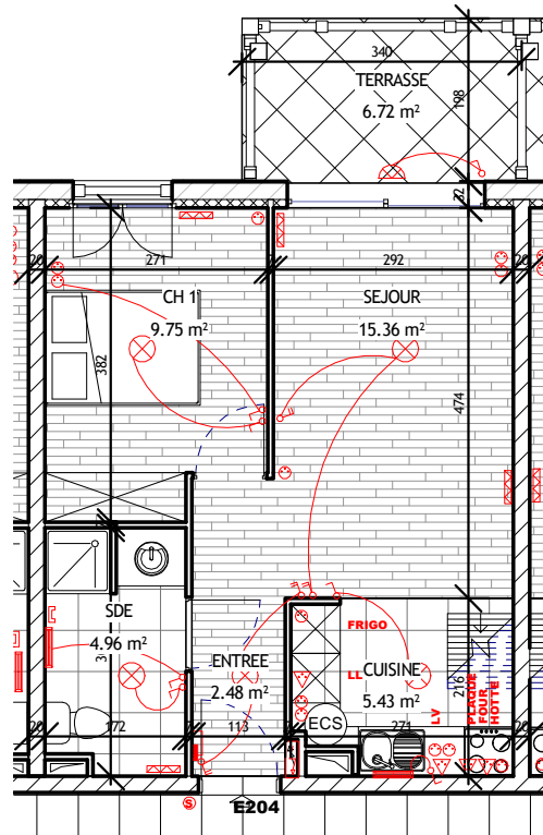
1 E 204 Ech : 1 : 100
