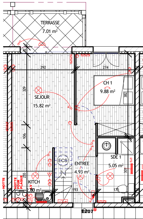
1 E 207 Ech : 1 : 100
