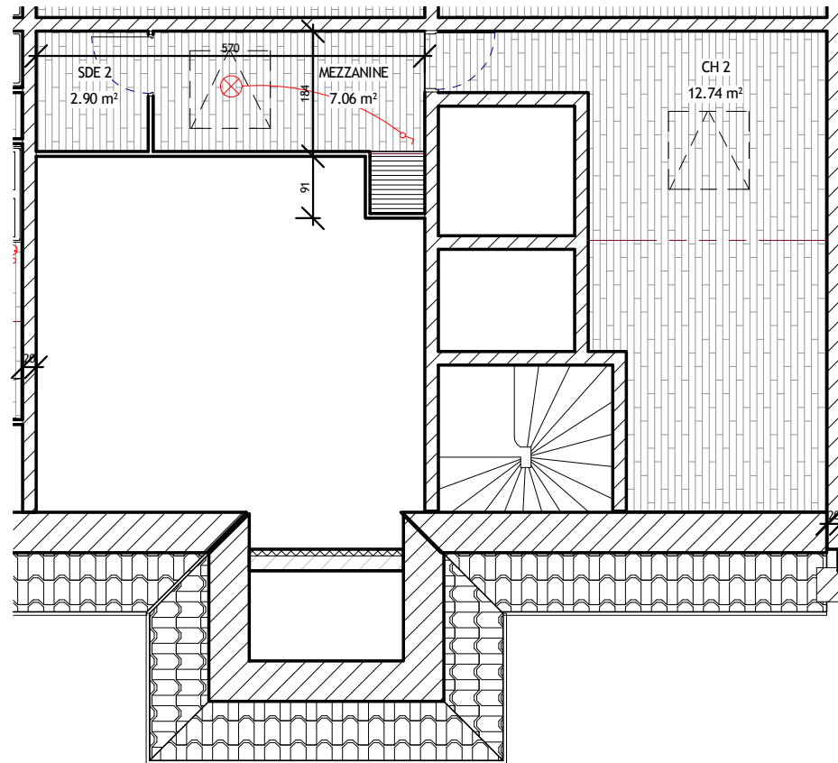
2 E301 Ech : 1 : 100
