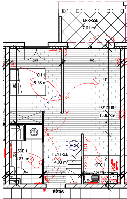
1 E 206 Ech : 1 : 100
