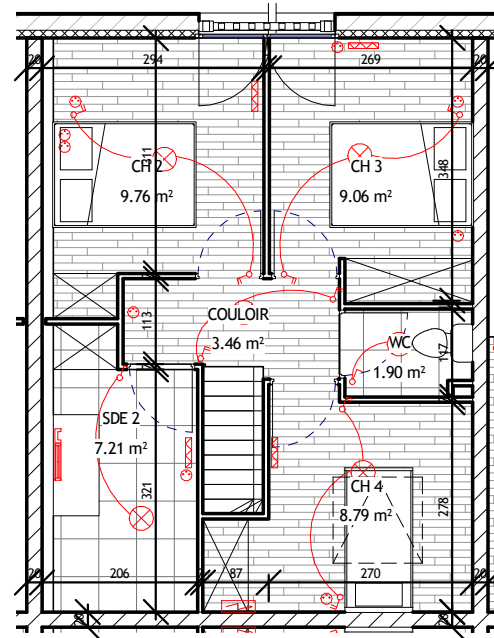
2 E307 Ech : 1 : 100
