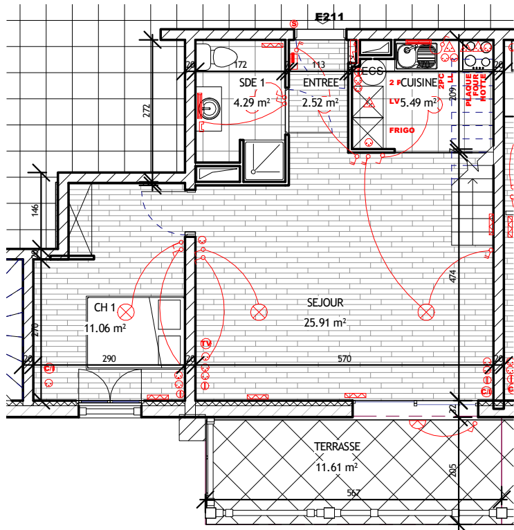
1 E 211 Ech : 1 : 100
